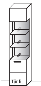
B 46,9 × H 207,0 × T 37,1 cm 5 Böden, 6 Fächer
