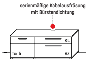
B 151,9 × H 55,8 × T 45,2 cm 1 Fach hinter Klappe, 2 Fächer hinter Tür
