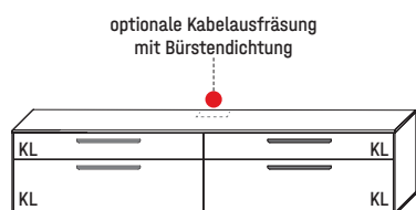
B 241,9 × H 53,8 × T 37,1 cm je 1 Fach hinter Klappen
