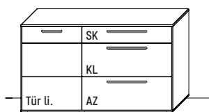
B 151,9 × H 89,4 × T 45,2 cm 1 Boden, 2 Fächer hinter Tür, 1 Fach hinter Klappe
