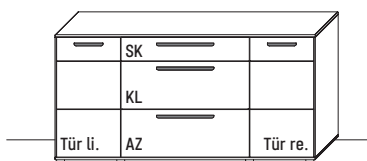
B 181,9 × H 89,4 × T 45,2 cm 2 Böden, 4 Fächer hinter Türen, 1 Fach hinter Klappe
