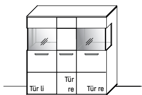
B 121,9 × H 123,0 × T 37,1 cm 9 Böden, 12 Fächer
