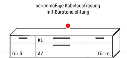
B 241,9 × H 55,8 × T 45,2 cm 1 Fach hinter Klappe, 4 Fächer hinter Türen
