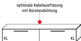
B 211,9 × H 37,0 × T 37,1 cm je 1 Fach hinter Klappen
