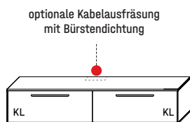
B 181,9 × H 37,0 × T 37,1 cm je 1 Fach hinter Klappen
