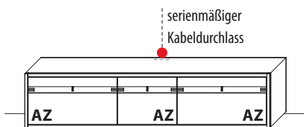
B 246,4 cm x H 56,4 cm x T 46,1 cm (serienmäßiger Vollauszug) 1 fester Boden hinter Auszug mittig / Fach B 58,1 cm x H 14,8 cm x T 34,0 cm
